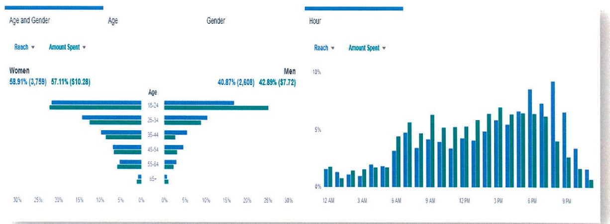
Facebook statistieken
